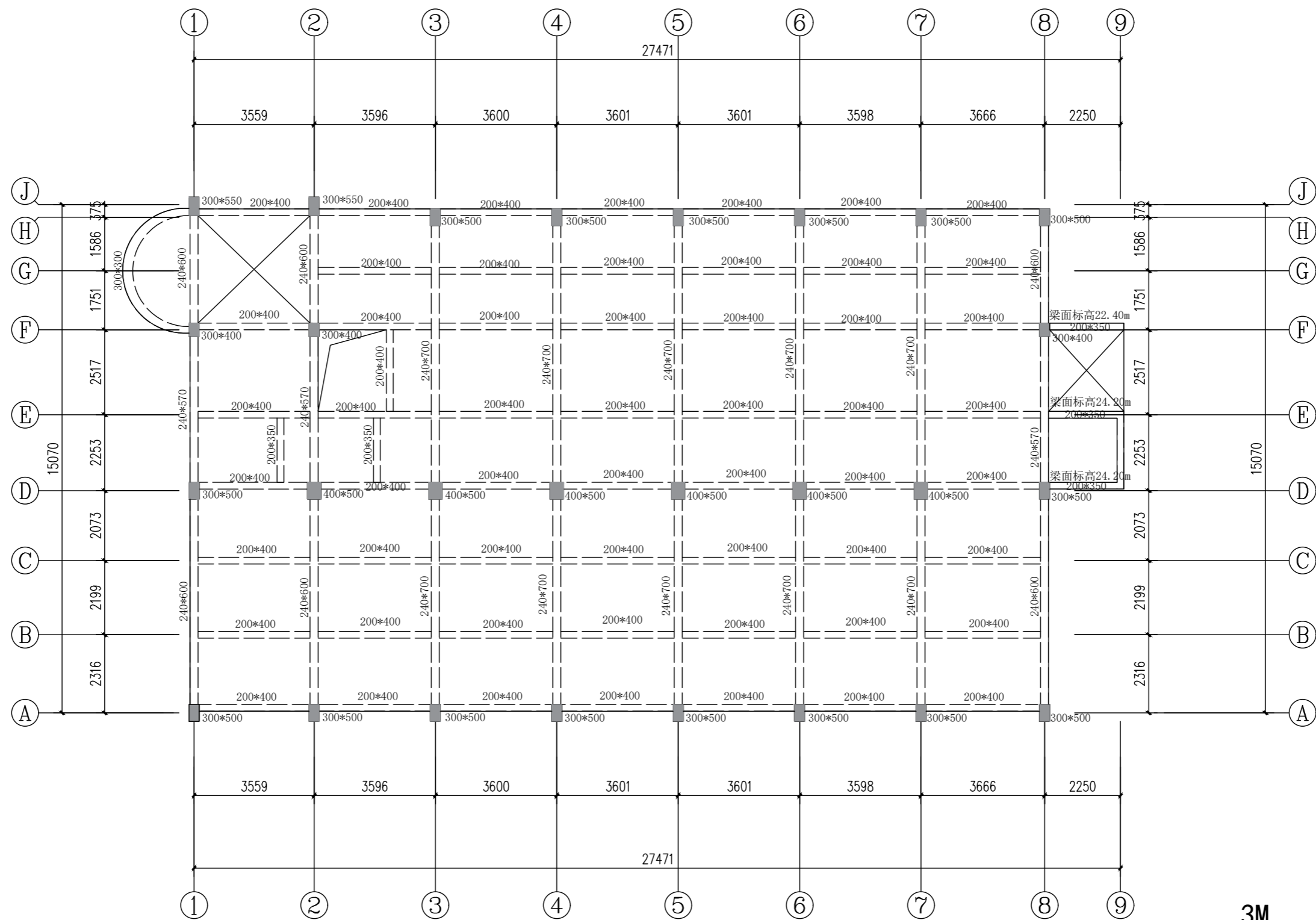
7层 (7层高3.50m, 楼板厚0.10m)
