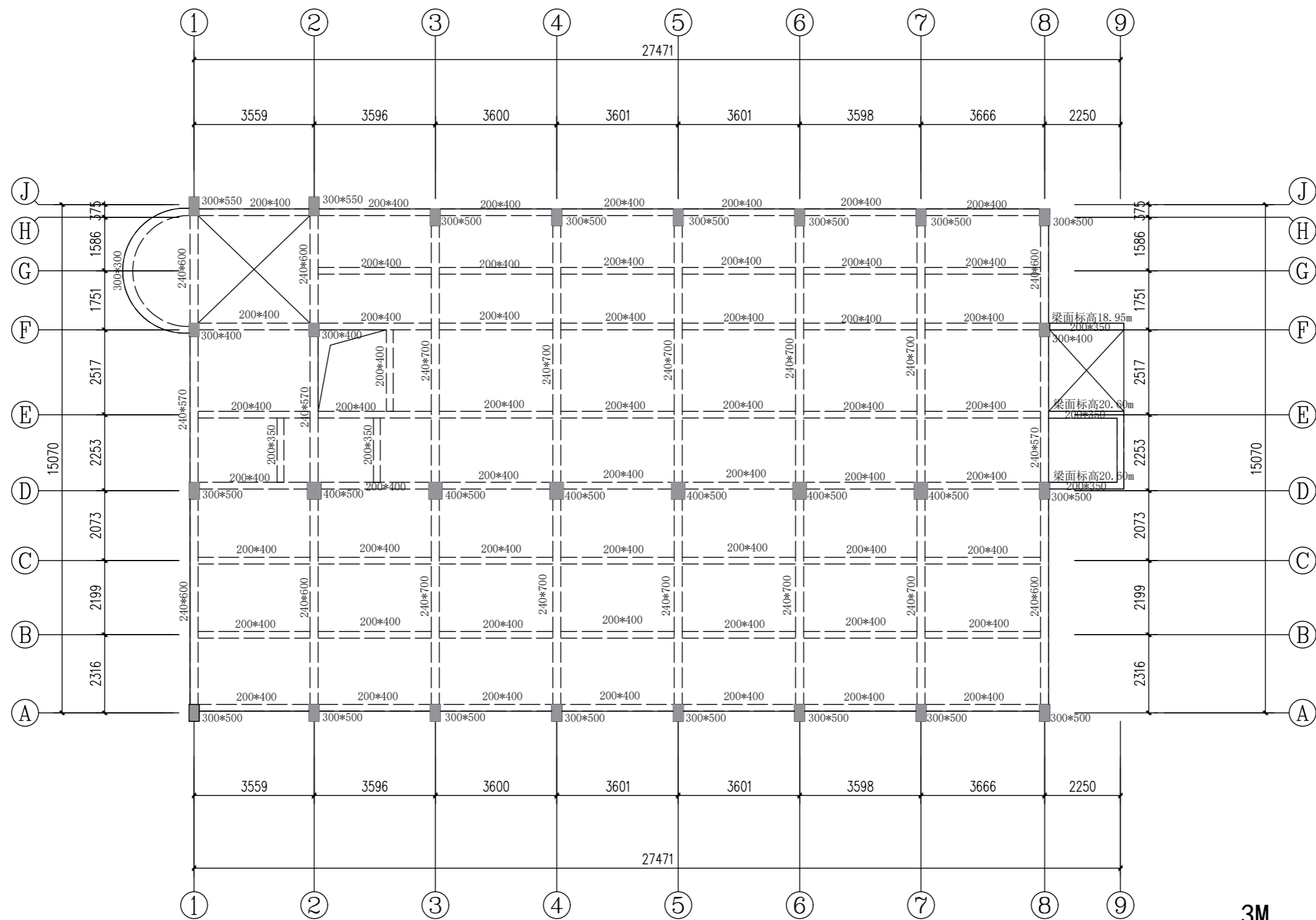
6层 (6层高3.20m, 楼板厚0.10m)
