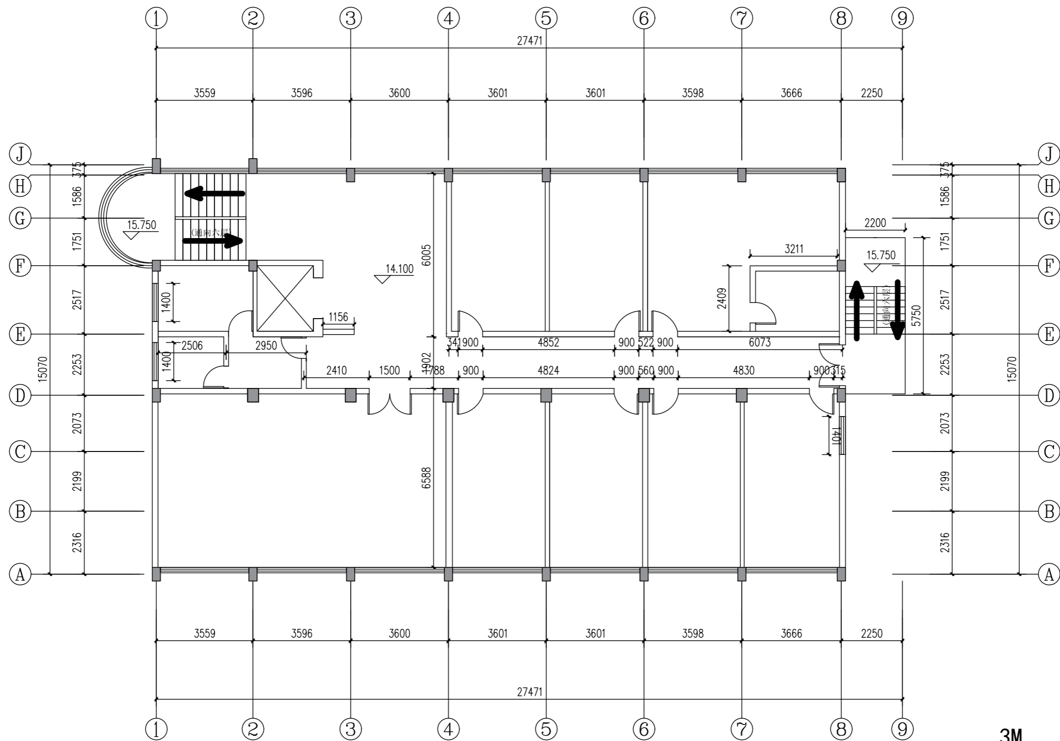
5层 (层高3.20m, 楼板厚0.10m)
