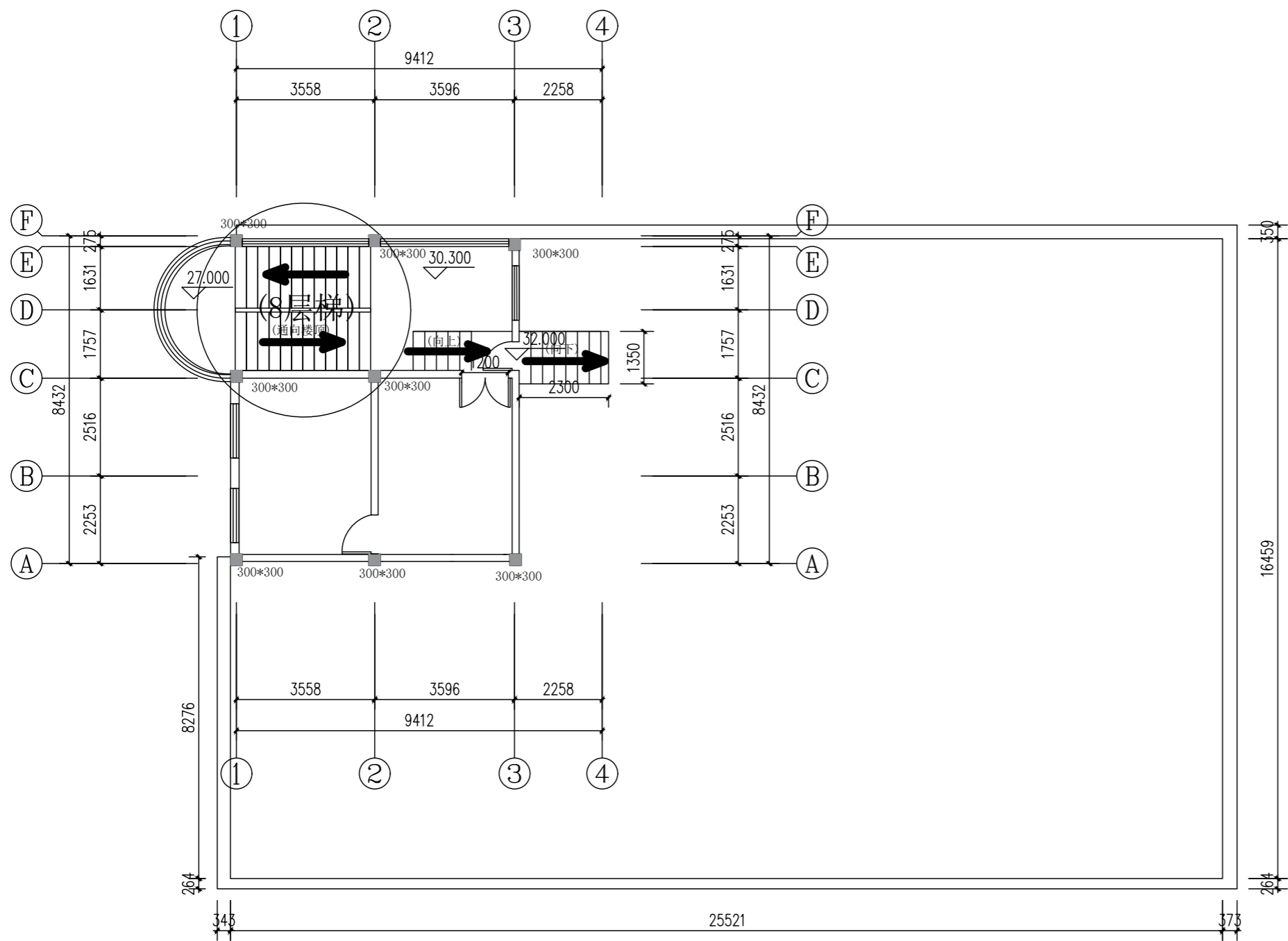
楼顶 (层高3.70m, 楼板厚0.10m)
