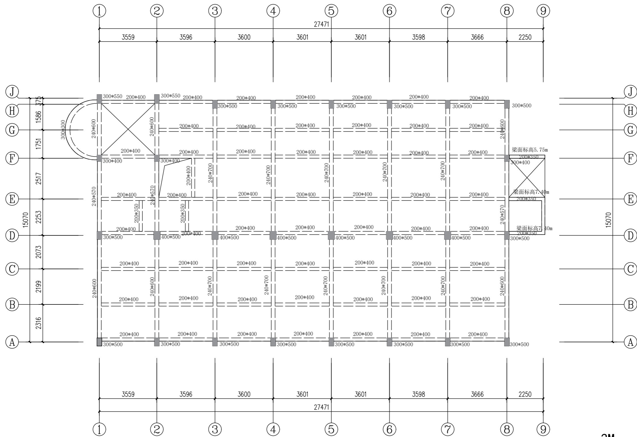
2层 (层高3.20m, 楼板厚0.10m)
