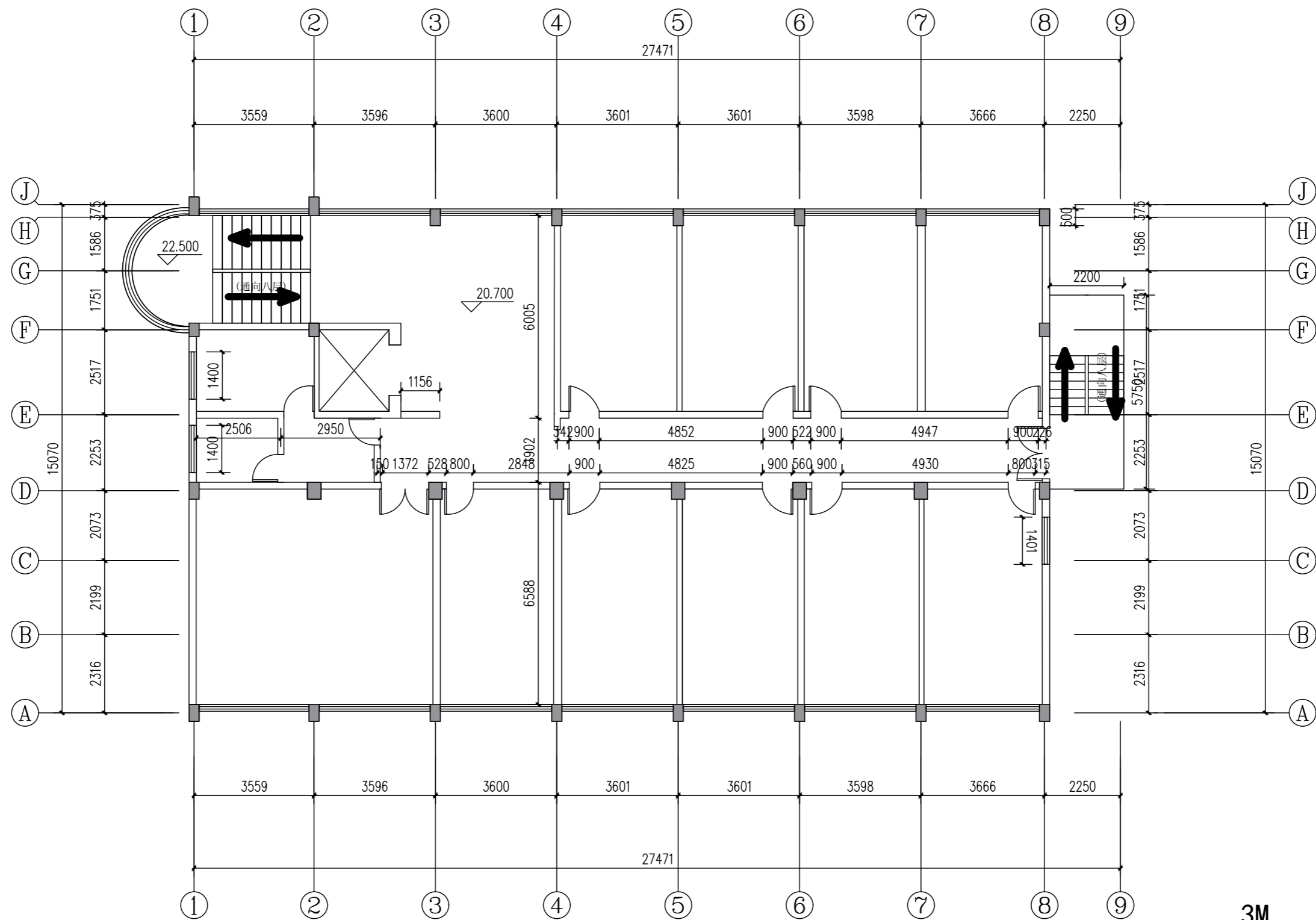
7层 (层高3.50m, 楼板厚0.10m)
