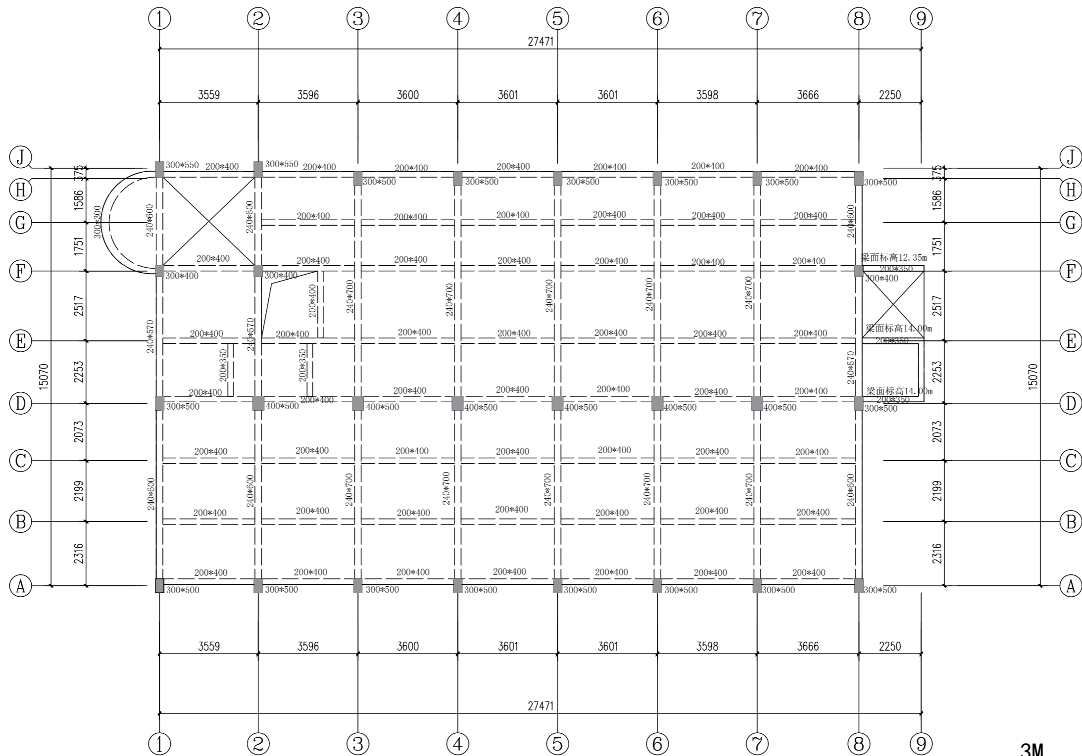
4层 (4层高3.20m, 楼板厚0.10m)
