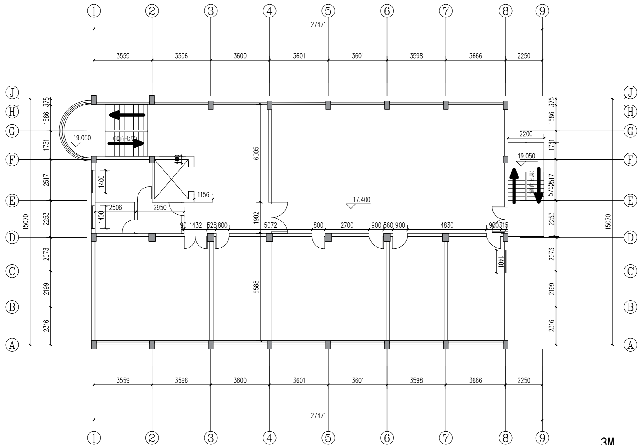
6层 (层高3.20m, 楼板厚0.10m)
