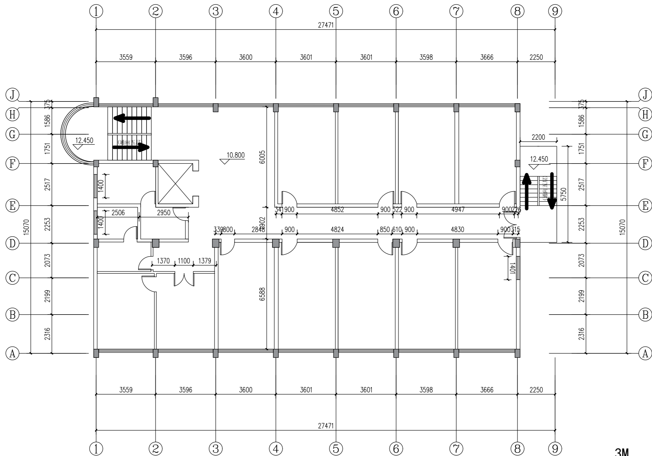
4层 (层高3.20m, 楼板厚0.10m)
