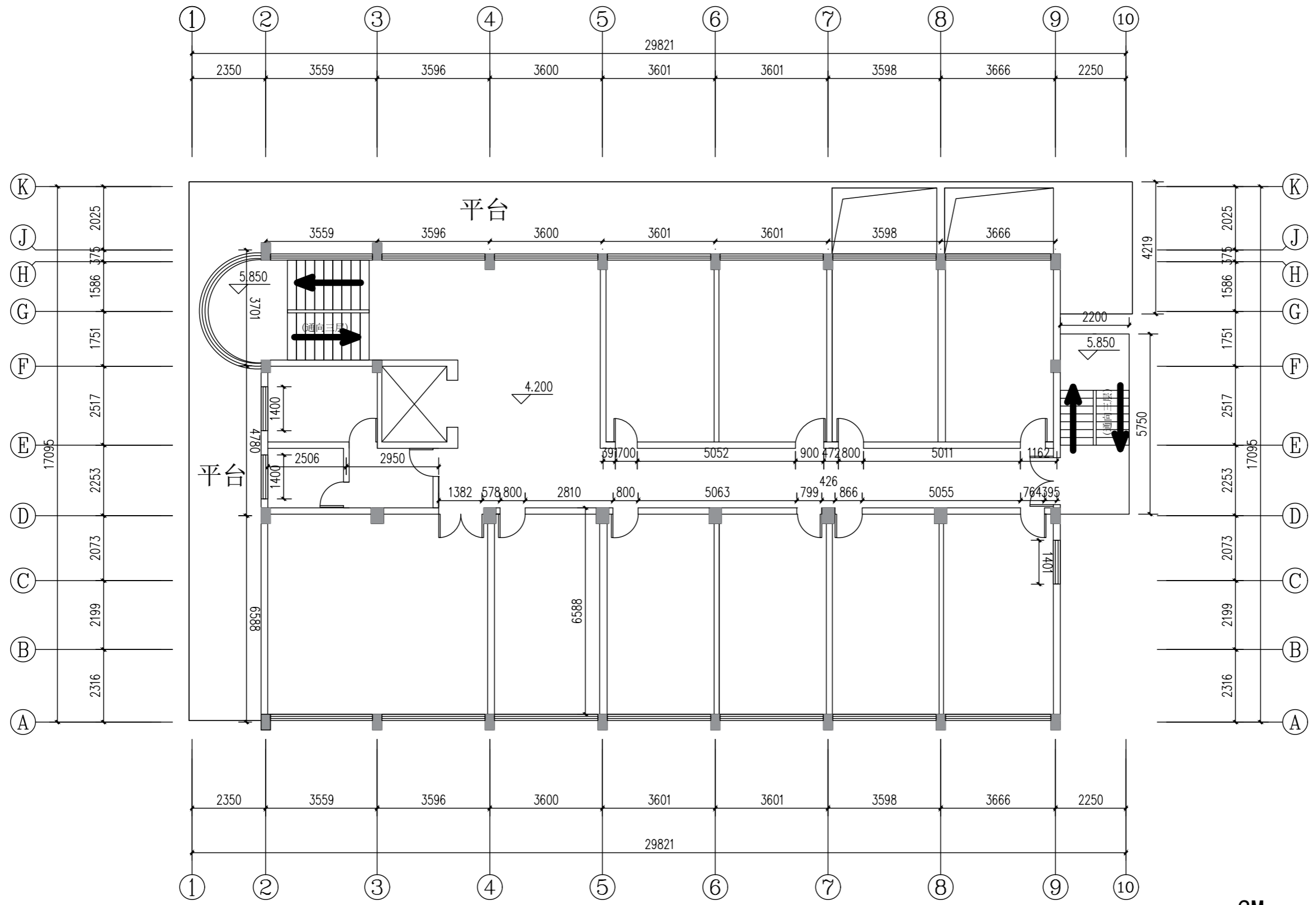
2层 (层高3.20m, 楼板厚0.10m)
