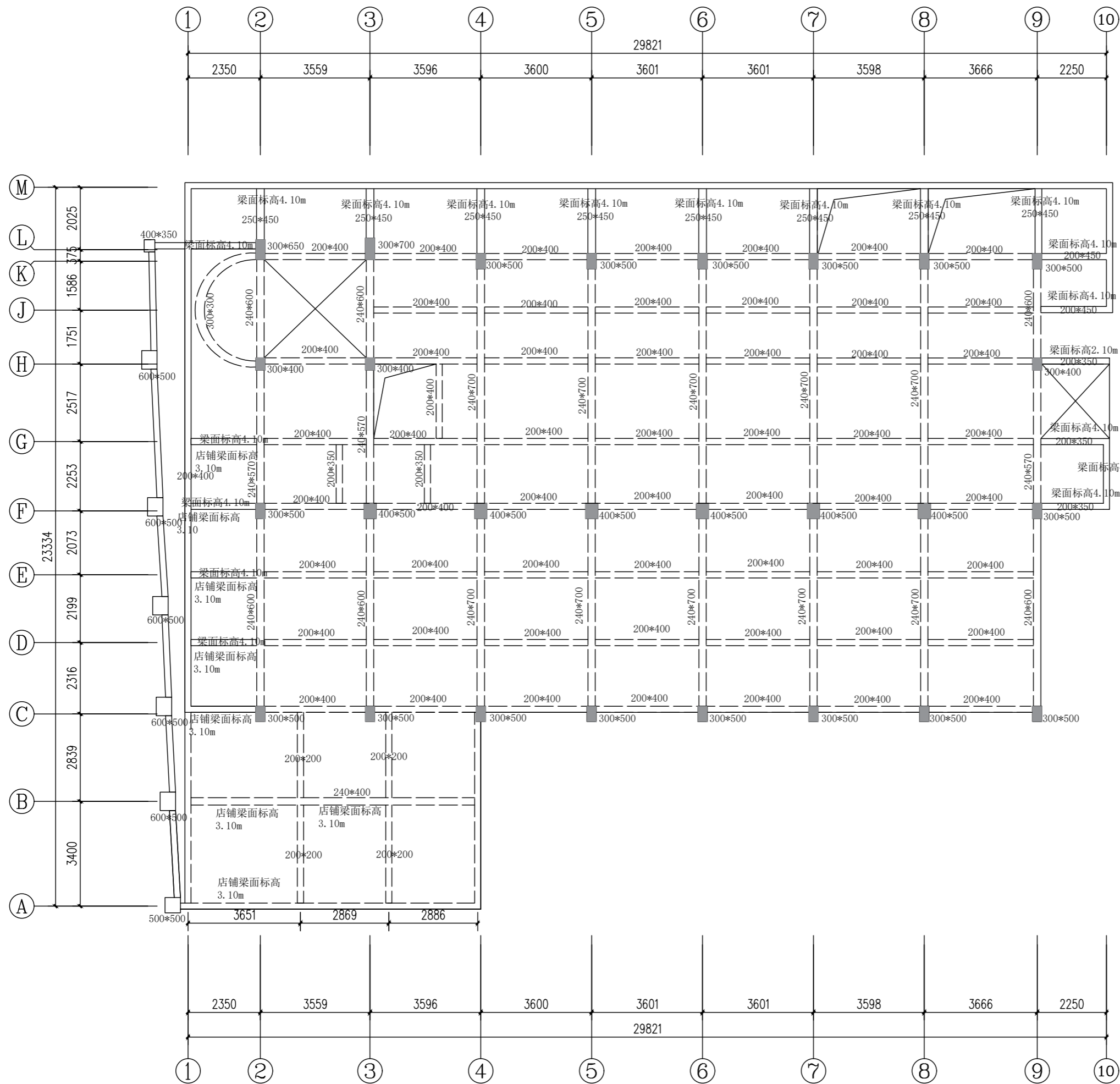
2层梁 (1层顶) (层高4.10m, 楼板厚0.10m) (标高以北侧一层大门为±0.00)
