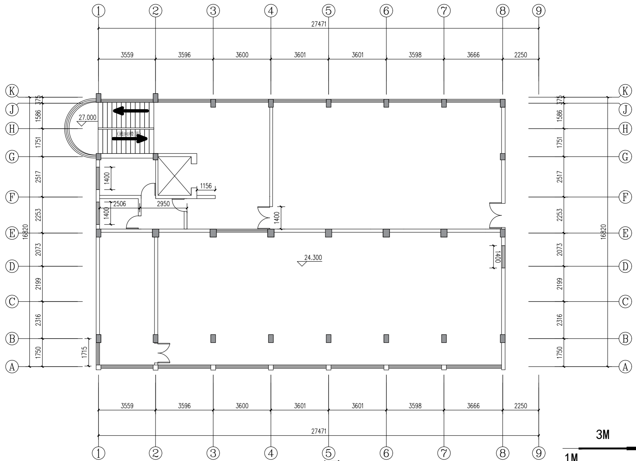
8层 (层高5.10m, 楼板厚0.10m)
